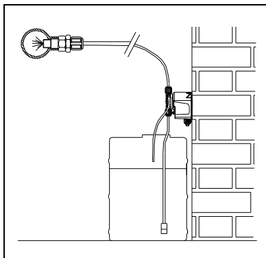
Рис.6 Монтаж на стене
