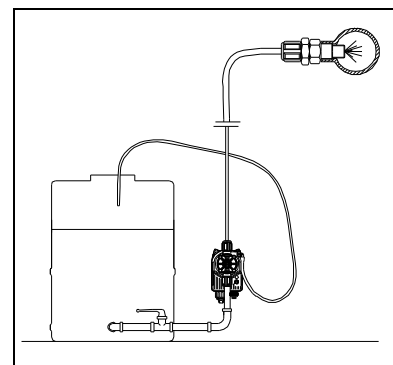
Рис.7: Монтаж на всасывающей трубе
