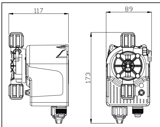
Рис.4 Габаритные размеры
