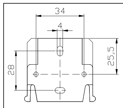
Рис.5 Шаблон для сверления
