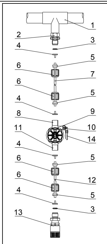
Рис. 8: Пример соединения
