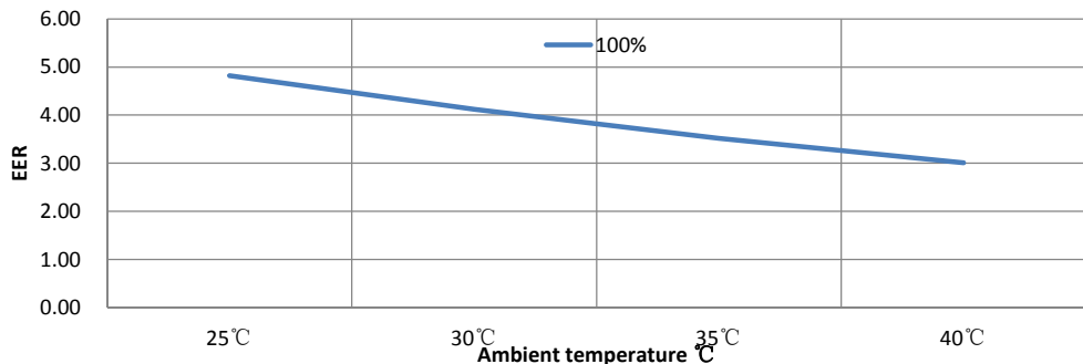
AXCR28 EER Curve
